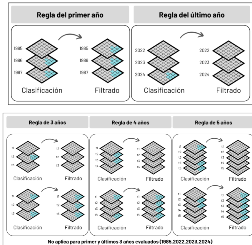
Figura 16. Filtro temporal
