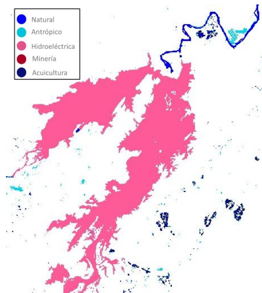
Figura 11. Ejemplo de categorías de cuerpo de agua. Fuente: elaboración propia.
