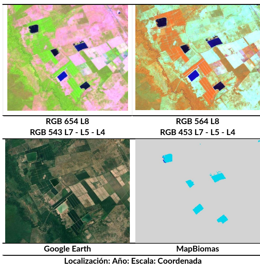
Figura 16. Respuesta espectral de la clase Otros cuerpos antrópicos. Fuente: elaboración propia.
