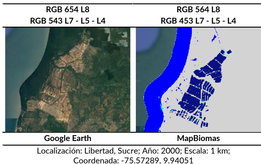
Figura 15. Respuesta espectral de la clase Acuicultura. Fuente: elaboración propia.
