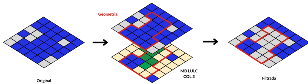
Figura 9. Funcionamiento de la limpieza adicional basada en geometrías y capas de referencia, donde se tomó la Colección 4 de MapBiomás Colombia (2025). Fuente: elaboración propia.
