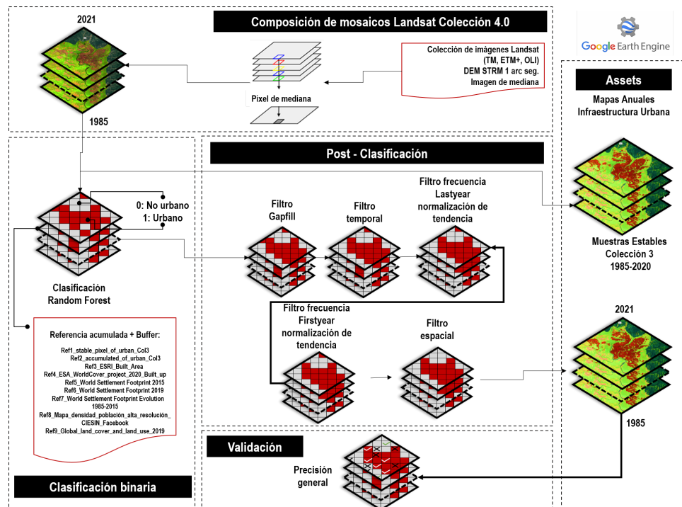
Figura 3. Flujo metodológico de la clasificación de Infraestructura Urbana Colección 1.0
