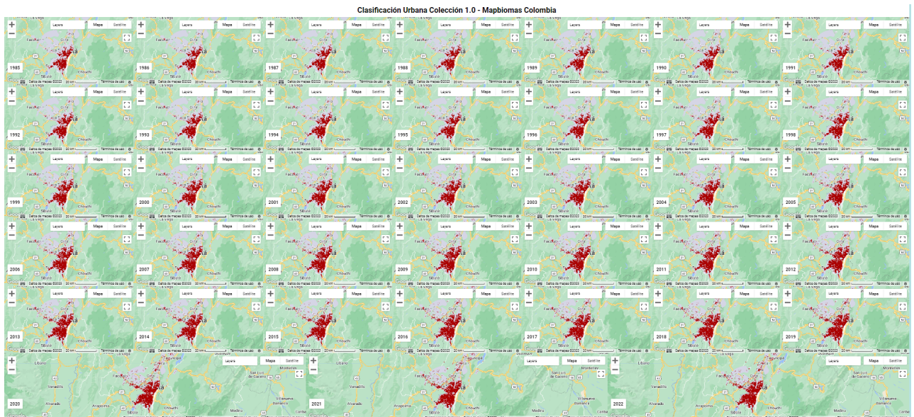
Figura 10. Clasificación multitemporal Infraestructura Urbana Colección 1.0 - 1985 a 2022 (caso Bogotá - Colombia).
